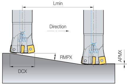
경사 가공
