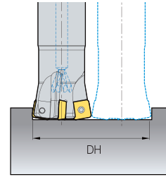
헬리컬 가공
